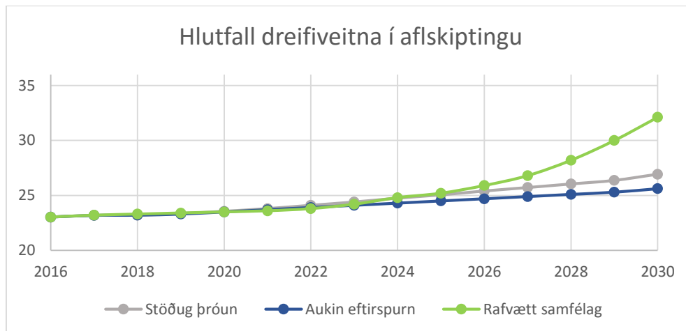
MYND 7-1 : HLUTFALL DREIFIVEITNA Í AFLSKIPTINGU
