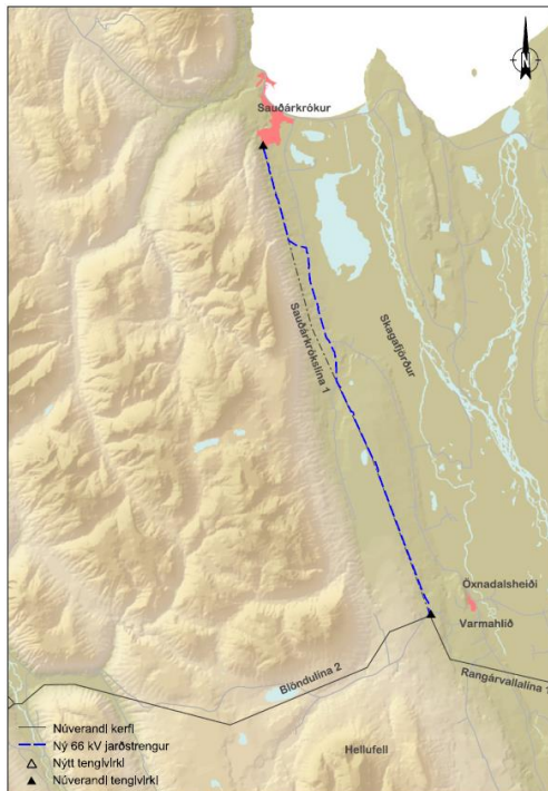
Mynd 5-13: Ný Sauðárkrókslína - Möguleg útfærsla nýs jarðstrengs
