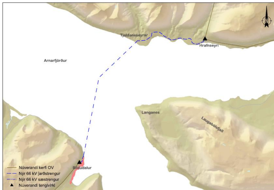
MYND 5-16 : MÖGULEGUR FYRSTI ÁFANGI STYRKINGAR Á SUNNANVERÐUM VESTFJÖRÐUM
