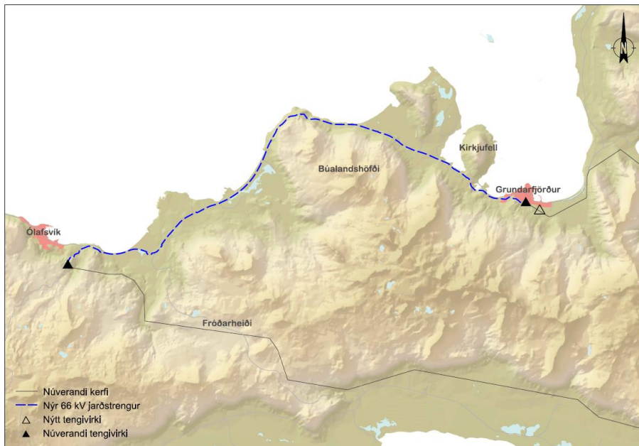
MYND 5-1: STAÐSETNING NÝS TENGIVIRKIS Í GRUNDARFIRÐI ÁSAMT GRUNDARFJARÐARLÍNU 2, SJÁ K. 5.2.6.
