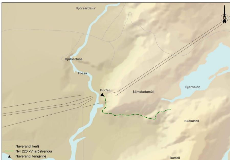
MYND 5-8: MÖGULEG ÚTFÆRSLA JARÐSTRENGS FRÁ BÚRFELLSVIRKJUN II.
