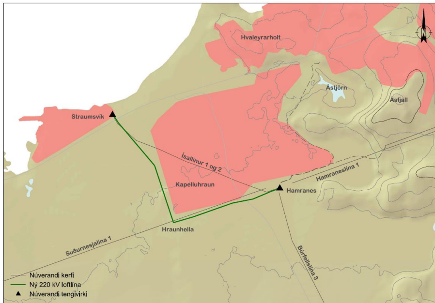
MYND 5-19 : LEGA ÍSALLÍNU 3
