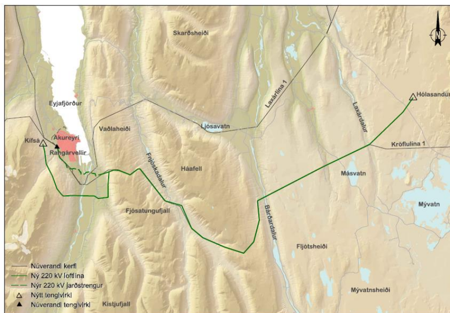
MYND 5-15: LÍNULEIÐ HÓLASANDSLÍNU 3.
