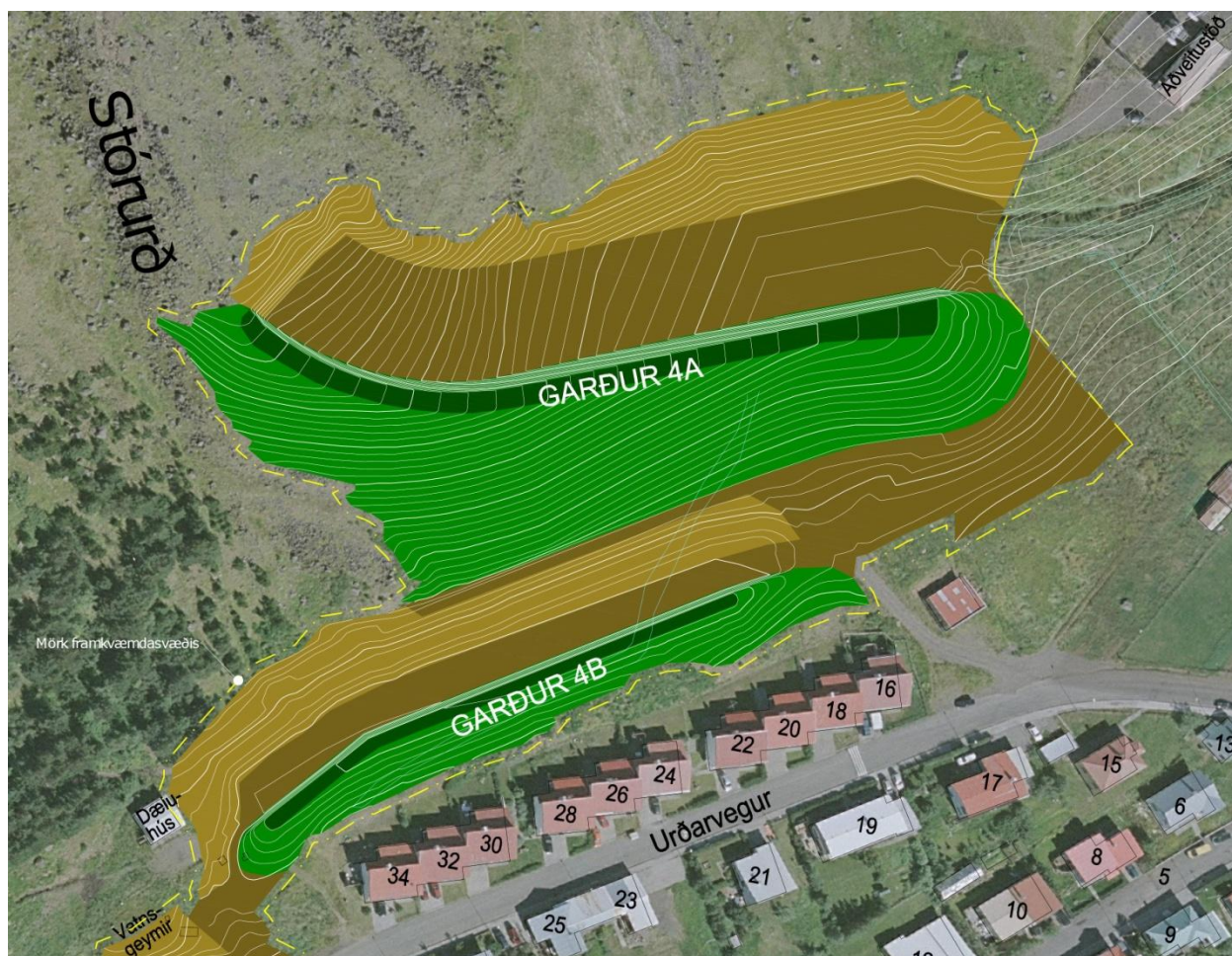
Mynd 3.4. Garður 4a og 4b, teiknað af Verkís. Sjá einnig teikningu 5 í viðhengi.
