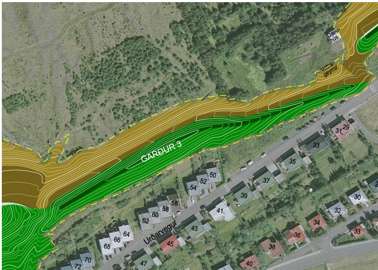
Mynd 3.3. Garður nr. 3, teiknað af Verkís. Sjá einnig teikningu 4 í viðhengi.
