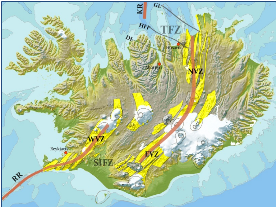
Mynd 21: Eldstöðvakerfi, gliðunar- og brotabelti 48
