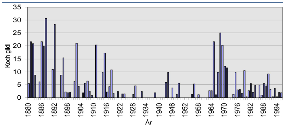
Mynd 23: Koch vísitala fyrir hafís við Ísland 1880-1996
