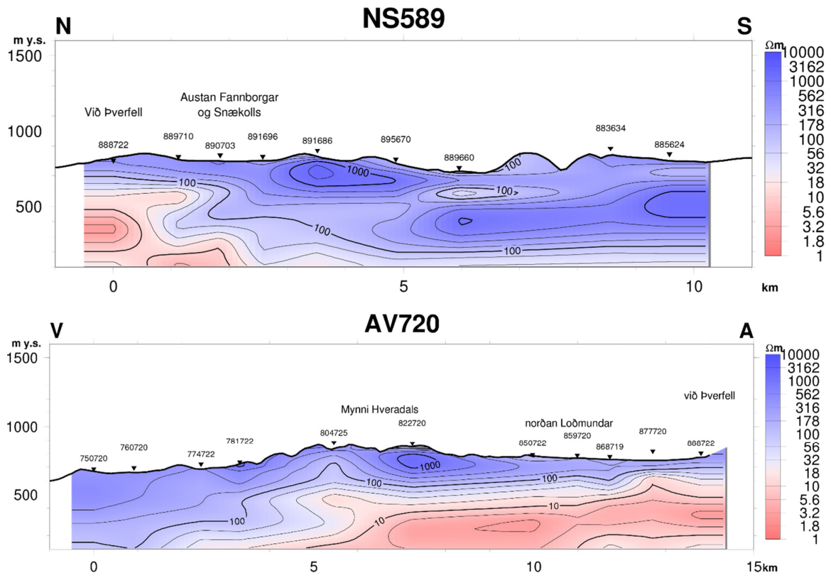
Mynd 4-3: Viðnámssnið af Þverfellssvæðinu (Ragna Karlsdóttir o.fl., 2010).
