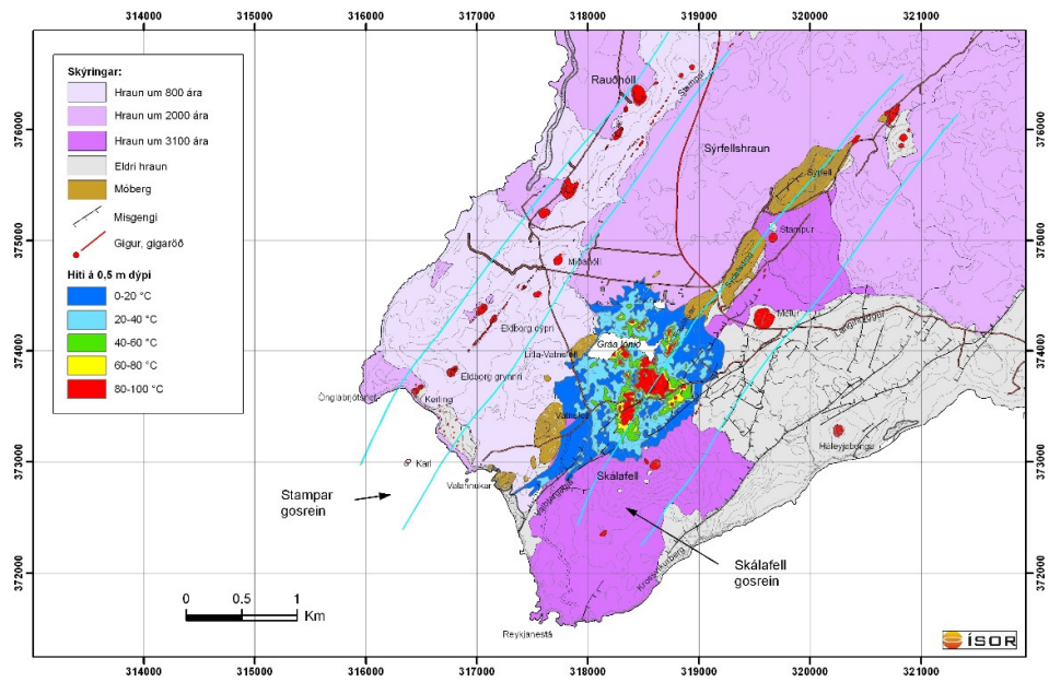
Mynd 4-1: Dæmi um háhitakerfi í snæðrekbelti (Jónas Ketilsson o.fl., 2010).
