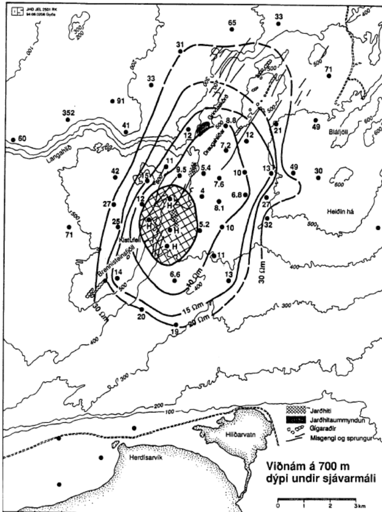
Mynd 4-3: Viðnámskort af Brennisteinsfjöllum (Ragna Karlsdóttir, 1995).
