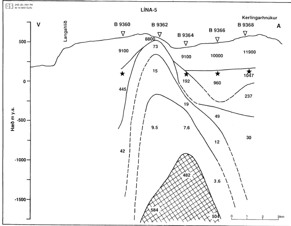
Mynd 4-4: Viðnámssnið af Brennisteinsfjöllum (Ragna Karlsdóttir, 1995).
