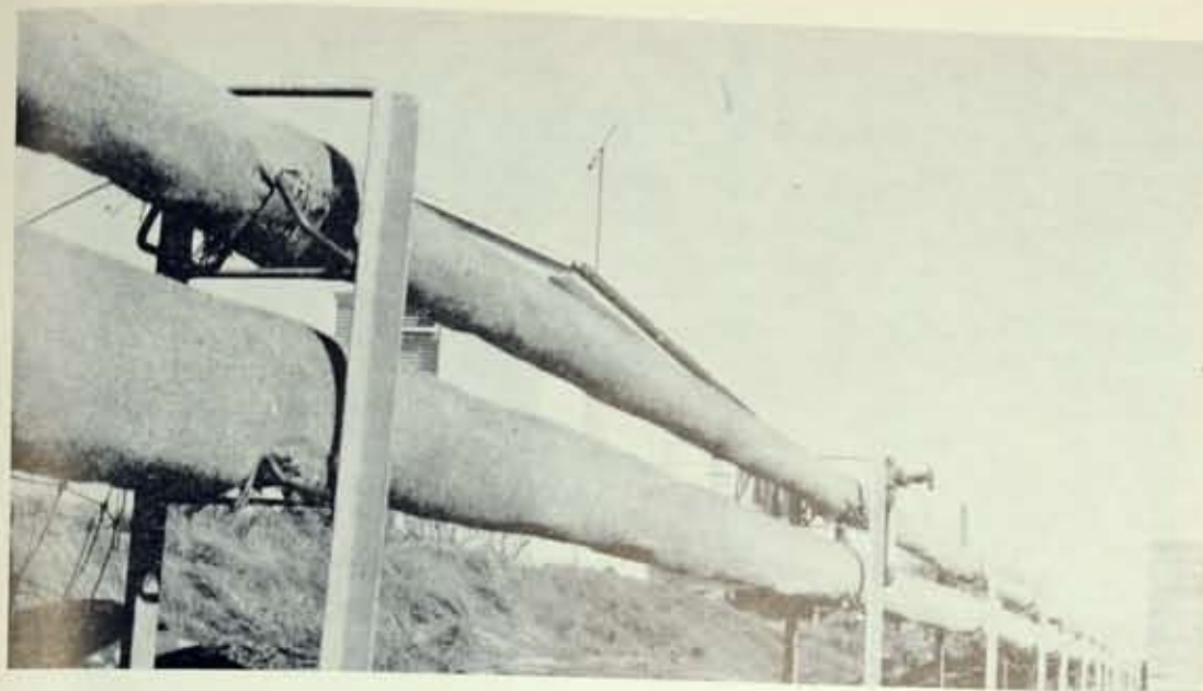
Kyndistöð fyrir Sigvaldahverfi og allmörg hús í nágrenninu tók til starfa í desember 1964. Þetta er fyrsti visir að hitaveitu í Kópavogi.
