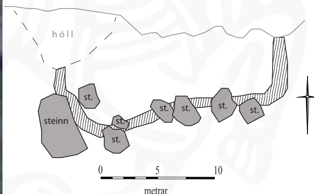
Rétt MH-108:050. Mynd til vinstri sýnir uppmælingu en teikning til hægri stikaða mælingu
