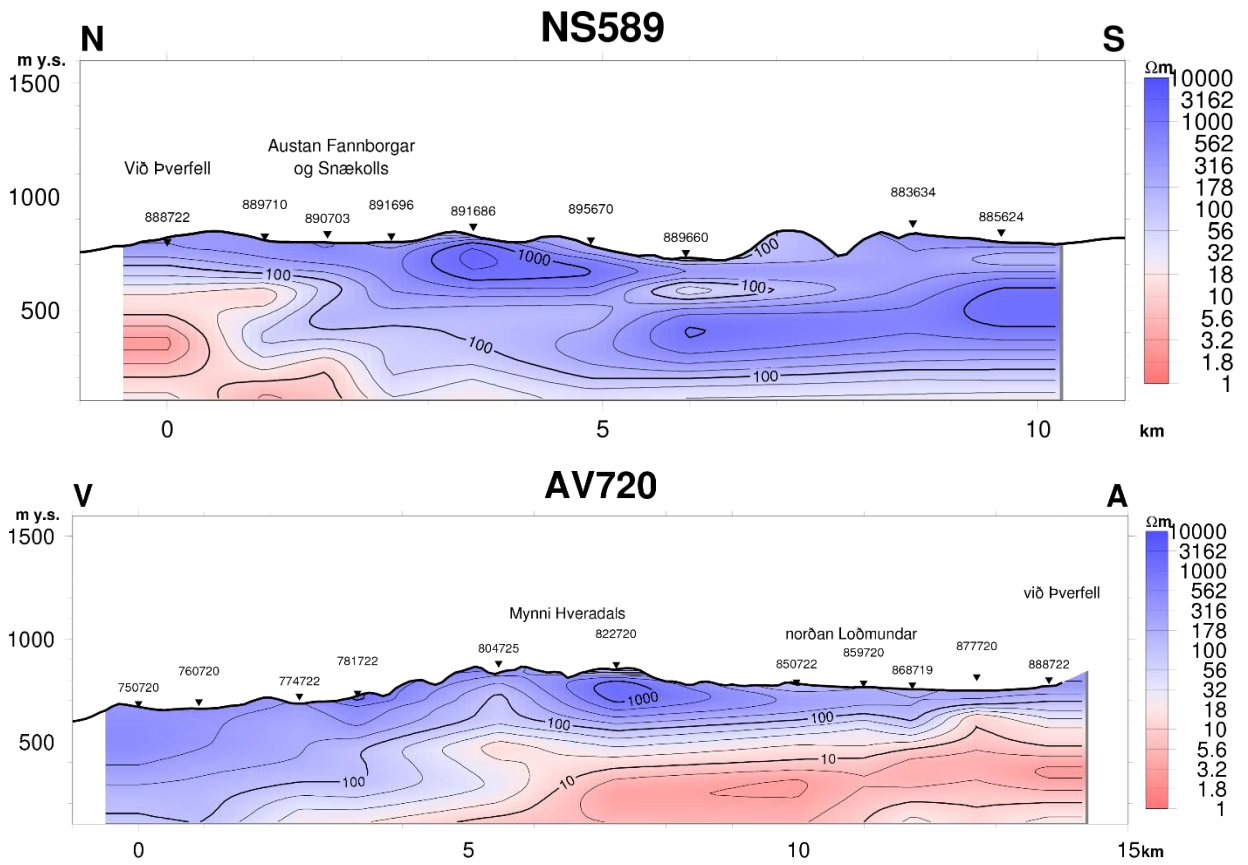
Mynd 4-3: Viðnámssnið af Þverfellssvæðinu (Ragna Karlsdóttir o.fl., 2010).
