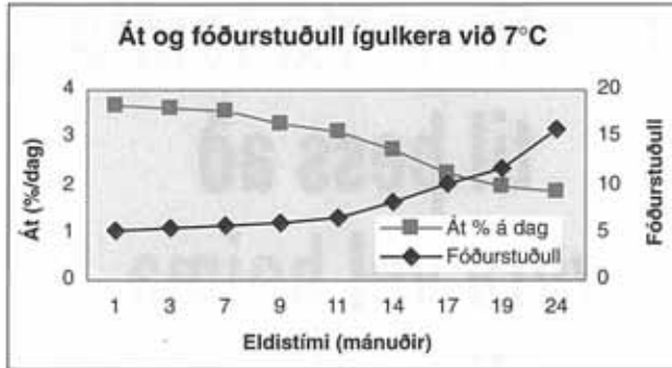
Mynd 2. Hlutfallslegt át og fódurnýting við 7°C.
